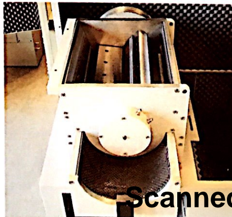
GRUPPO TESTA 600/25/MP360
