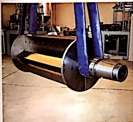
ROTORE 1000/100/P500
